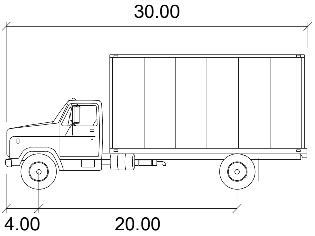
SU-30
