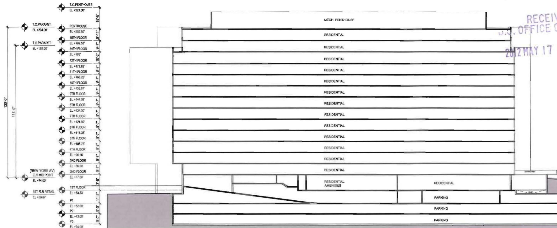
1 Section A-A
