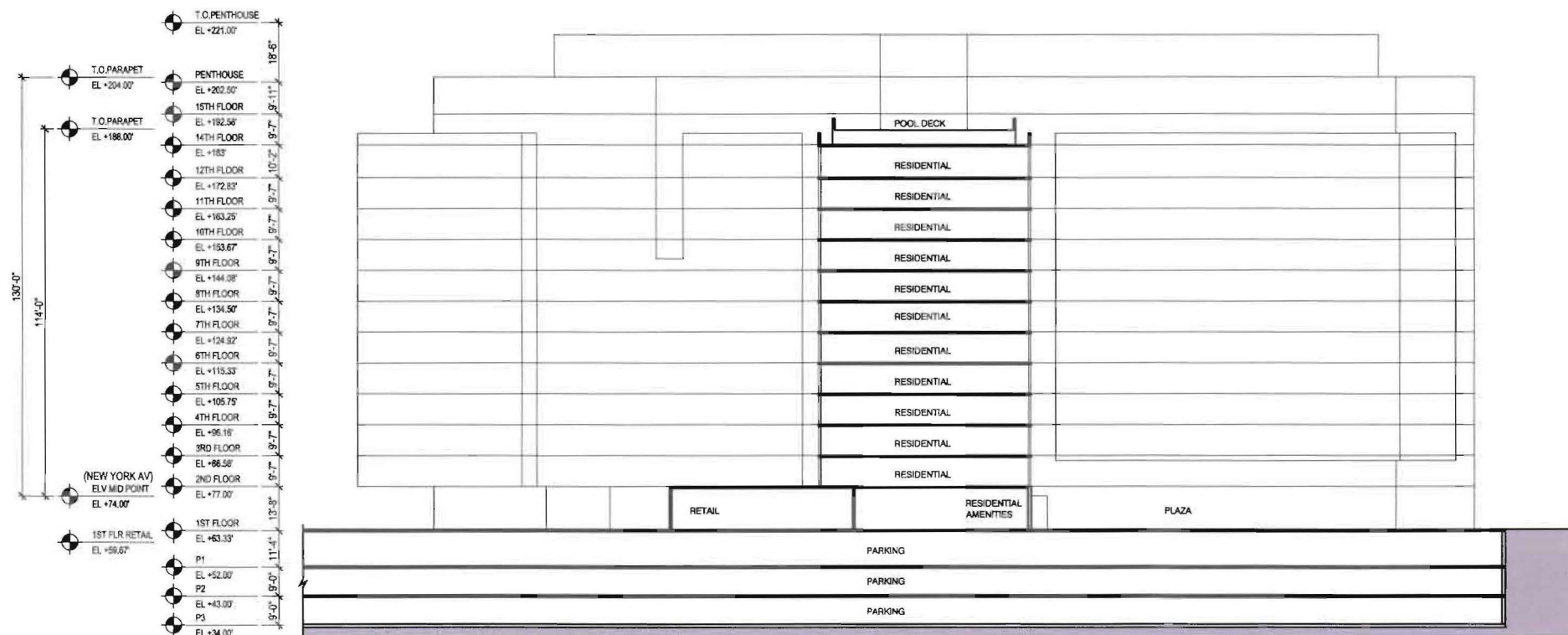
1 Section A-A
