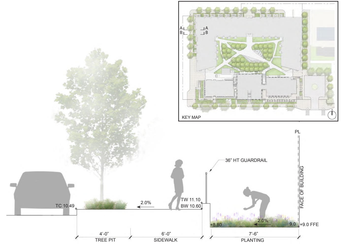
SECTION A-A
