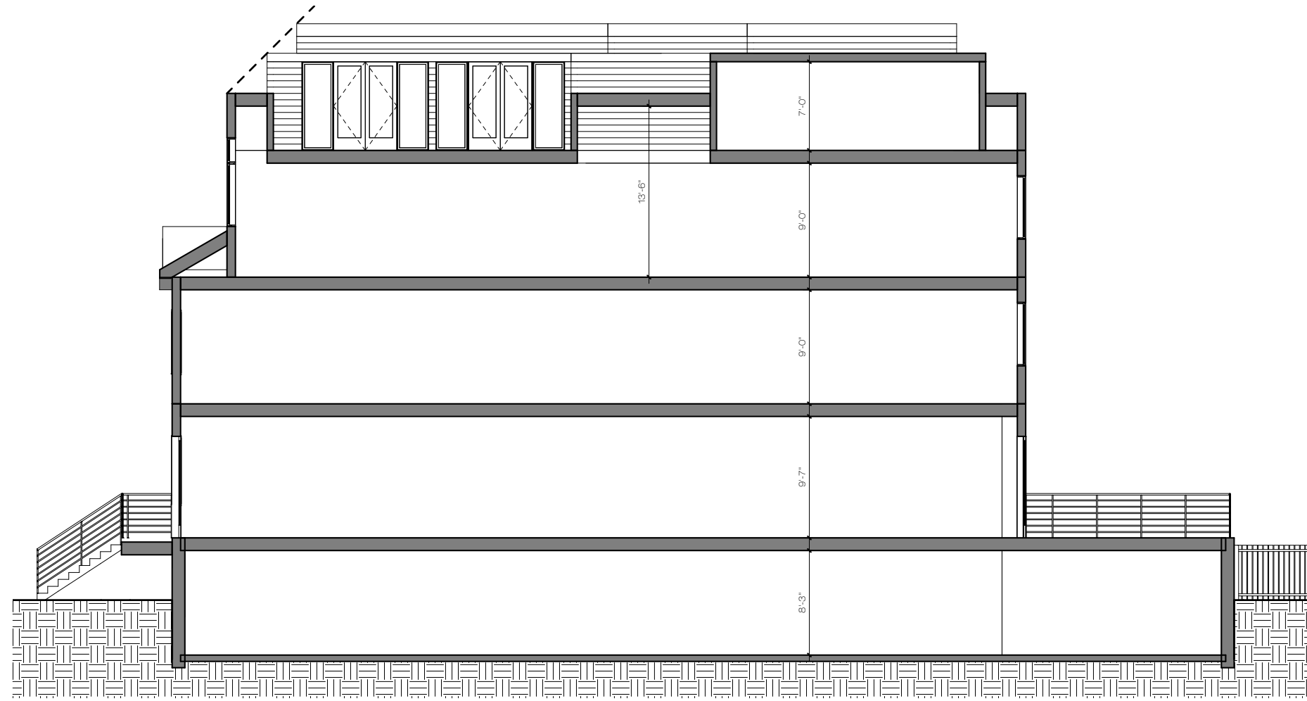
② LONGITUDINAL SECTION 2
