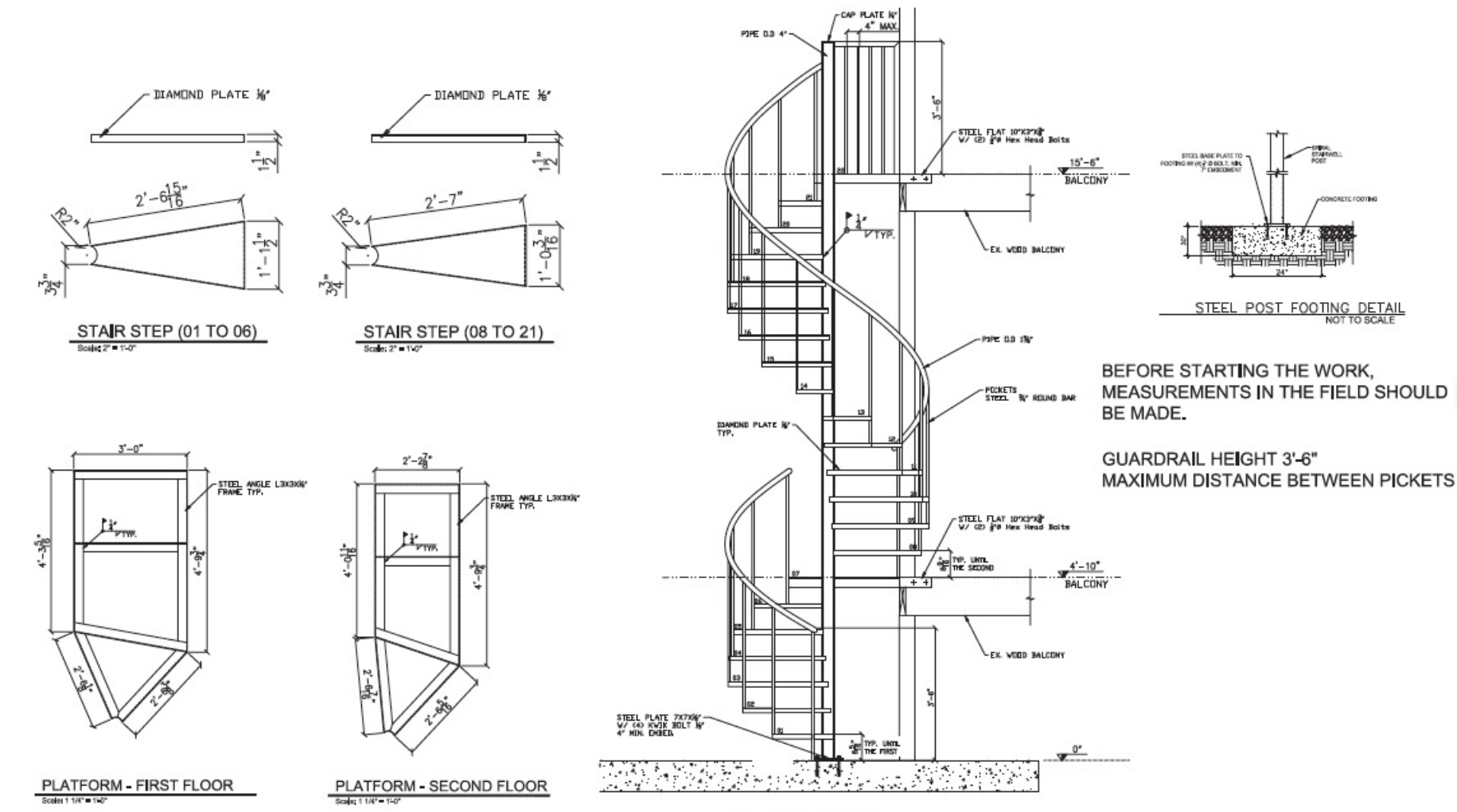
SECTION MD02 Scale: 1/4" = 1'-0"
