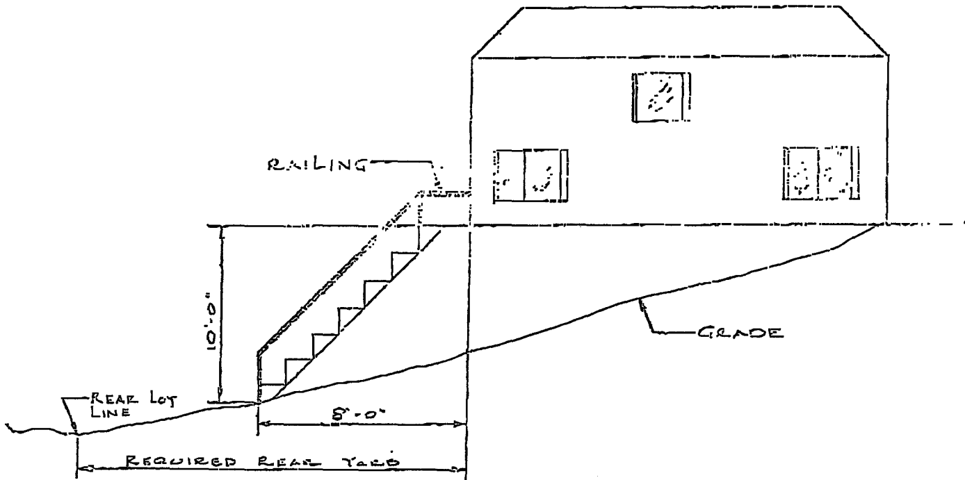
ELEVATION N.T.S.
