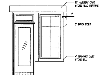
8 A-501 DOOR TYPE #8 Scale: 3/16"=1'-0"
