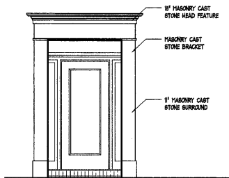
2 A-501 DOOR TYPE #2 Scale: 3/16"=1'-0"
