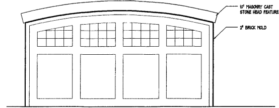
12 A-501 DOOR TYPE #12 Scale: 3/16"=1'-0"
