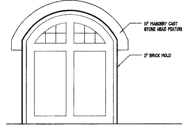
11 A-501 DOOR TYPE #11 Scale: 3/16"=1'-0"
