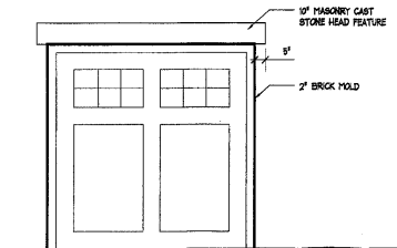
10 A-501 DOOR TYPE #10 Scale: 3/16"=1'-0"
