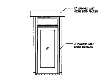
4 A-501 DOOR TYPE #4 Scale: 3/16"=1'-0"
