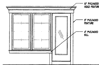
9 A-501 DOOR TYPE #9 Scale: 3/16"=1'-0"
