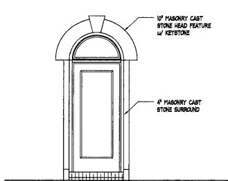
3 A-501 DOOR TYPE #3 Scale: 3/16"=1'-0"
