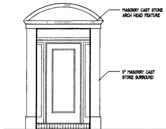
6 A-501 DOOR TYPE #6 Scale: 3/16"=1'-0"
