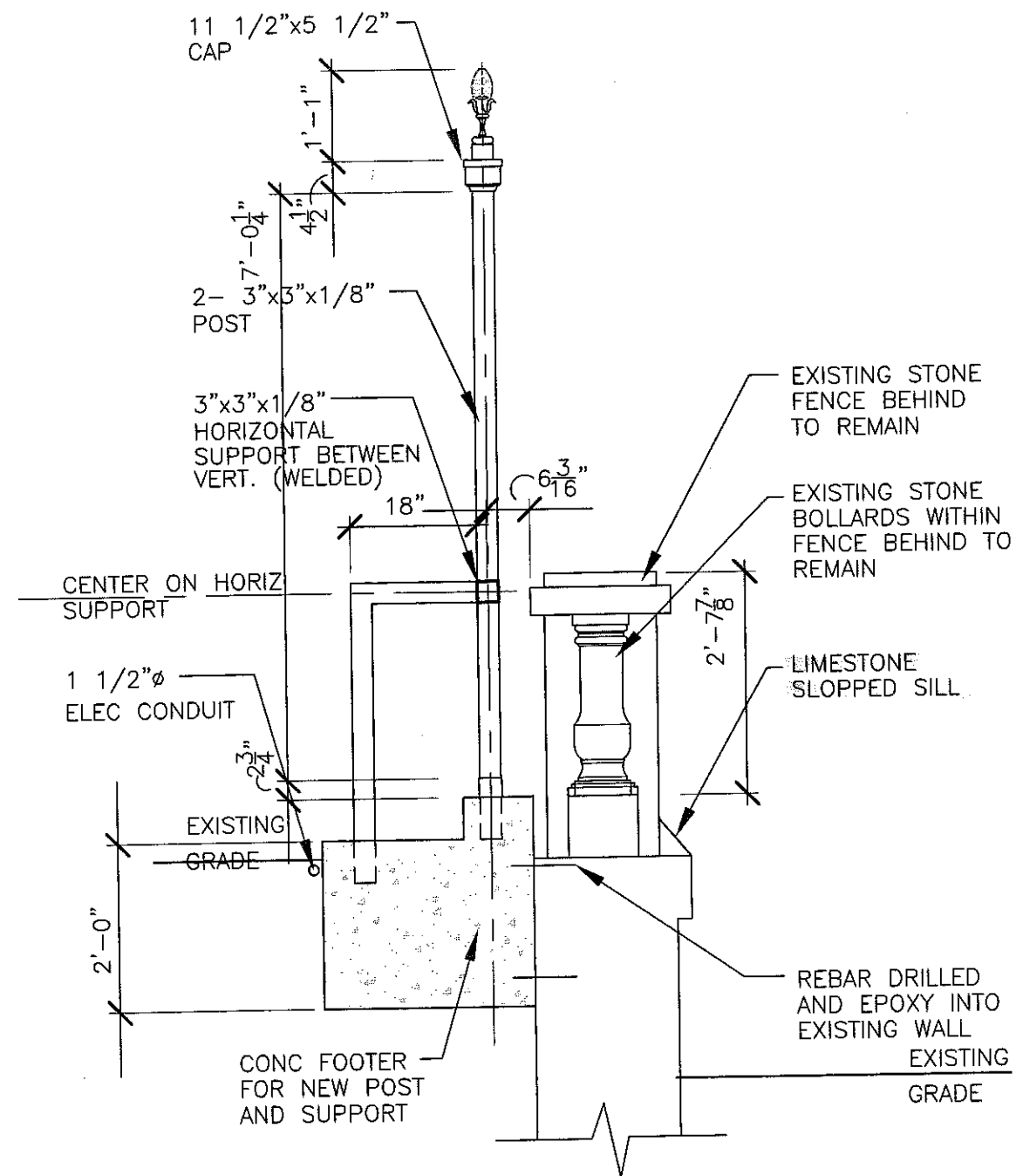
02 POST/FENCE SECTION SCALE: 1/2"=1'-0"
