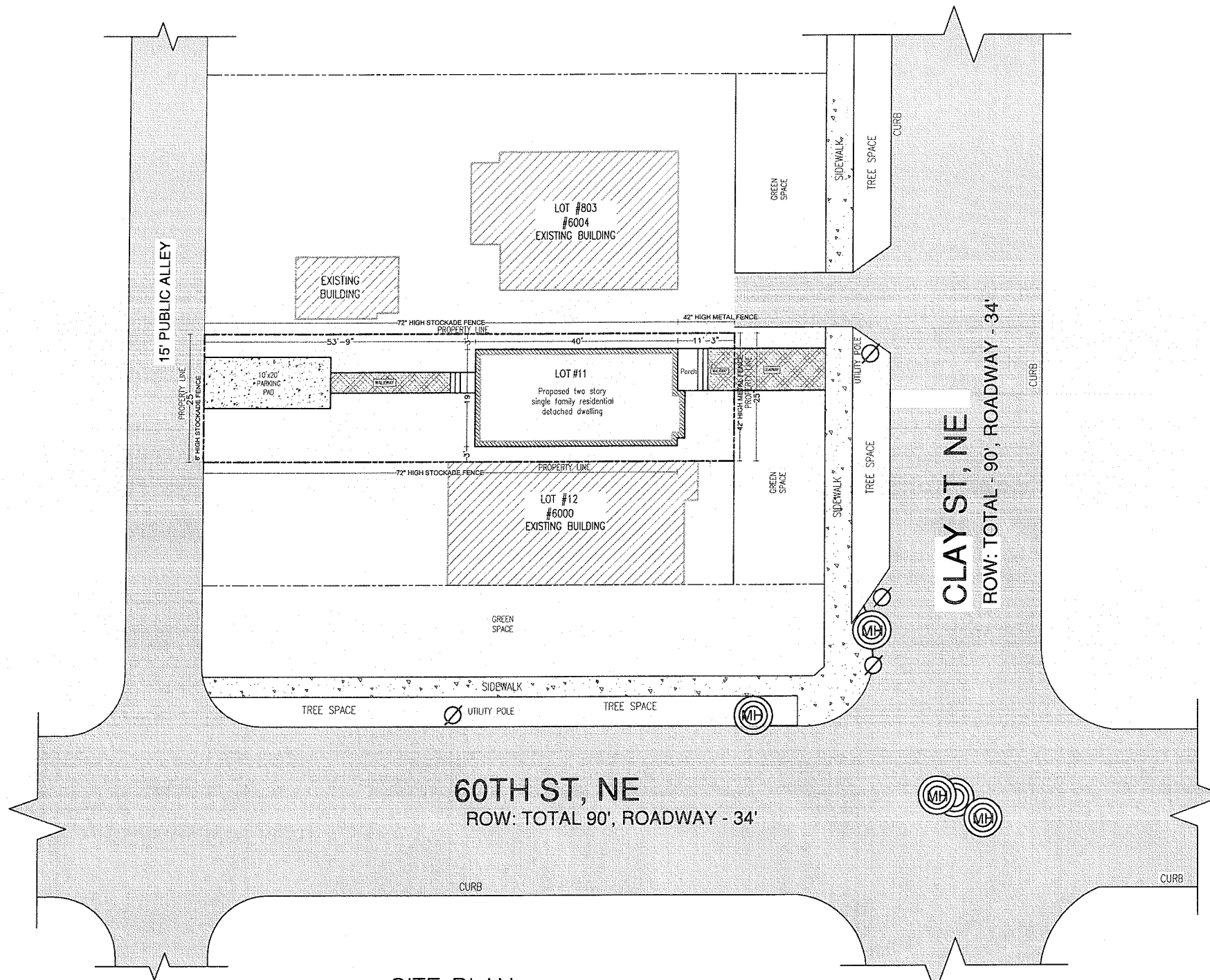
SITE PLAN 6002 CLAY ST NE
