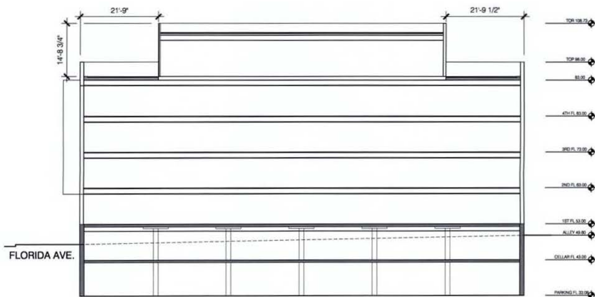
LONGITUDINAL SECTION 1/16" = 1'-0"
