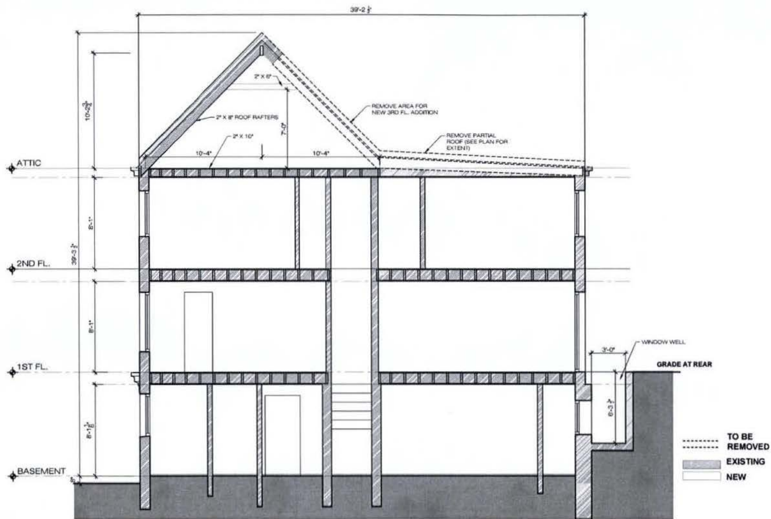
01 EXISTING LONGITUDINAL SECTION SCALE: 3/16" = 1'-0"
