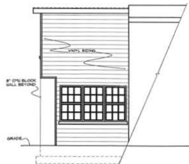
RIGHT ELEVATION
