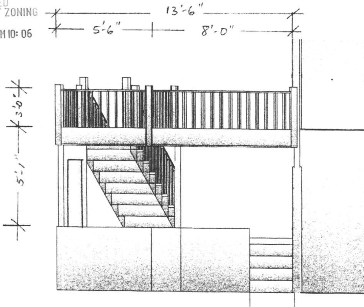
RIGHT ELEVATION
